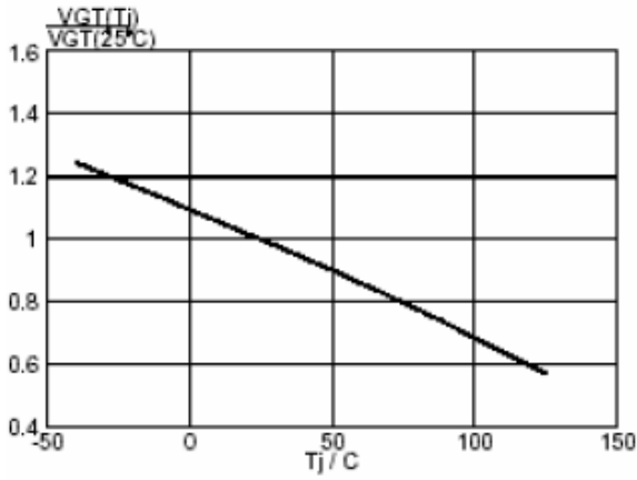
图 7: V_{GT} 与结温关系
