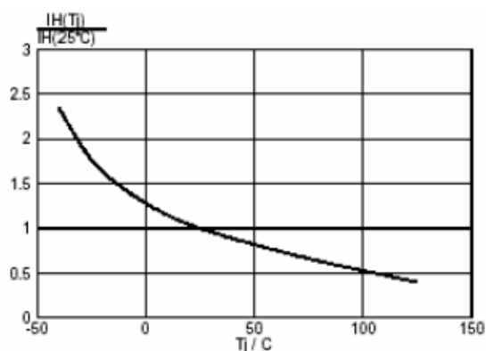
图 3: I_H 与结温关系
