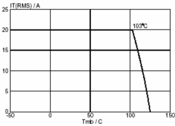
图 5: I_{T(RMS)} 与温度关系
