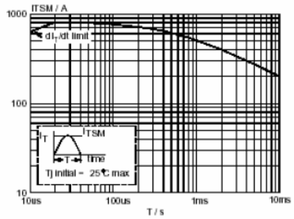
图 10: I_{TSM} 与导通时间关系
