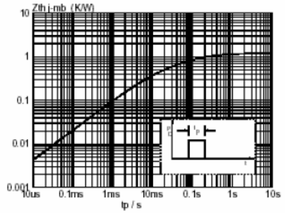
图 8: 温升与导通脉宽关系
