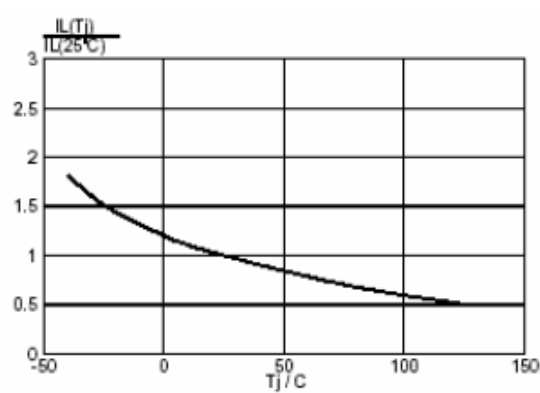
图 2: I_L 与结温关系
